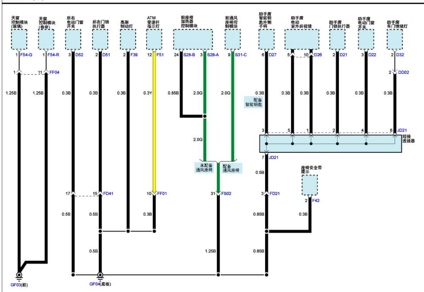
搭铁分布(11)
